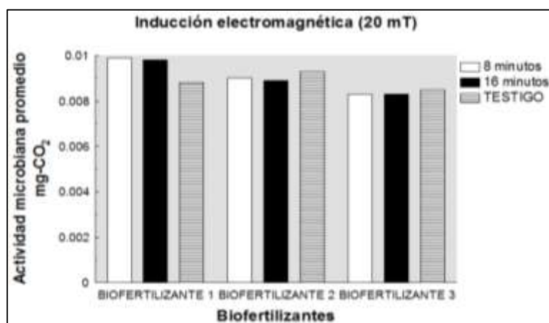
Figura 24 Resultados prueba de actividad microbiana de los tres (3) biofertilizantes para una inducción electromagnética de 20 mT.
