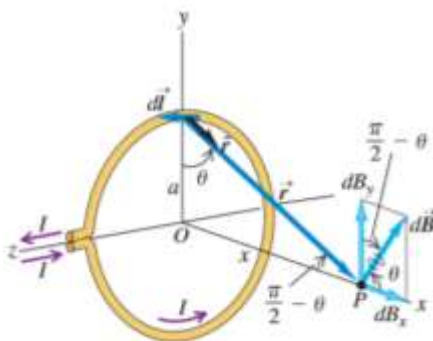
Figura 5 Campo magnético de una espira circular con corriente.
