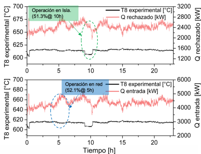
Figura 6: Comparación entre predicción del modelo propuesto para T8 y el calor rechazado y calor de entrada del gas natural.
