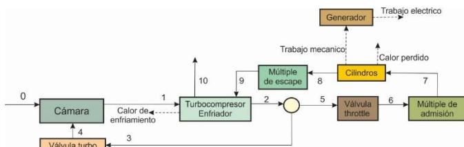
Figura 2: Sistema de diagrama de proceso. Fuente: Elaboración propia.
