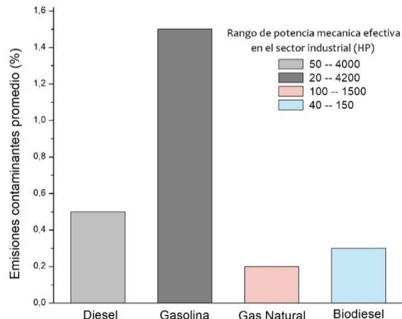
Figura 1: Rango de potencia y emisiones de motores de generación por combustible.
