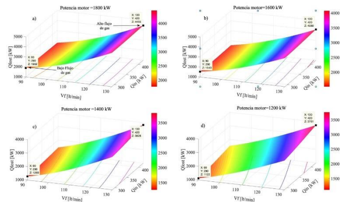
Figura 4: Caracterización de la transferencia de calor en los cilindros del motor J612 Jenbacher a diferentes potencias, a) 1.8 MW, b) 1.6 MW, c) 1.4 MW y d) 1.2 MW.
