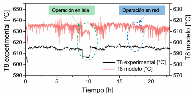
Figura 5: Comparación entre la predicción del modelo propuesto para T8 y los valores experimentales.
