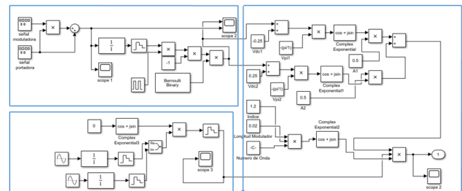
Figura 2: Diagrama de bloques desarrollada en la herramienta computacional, para la etapa de las señales de entrada.
